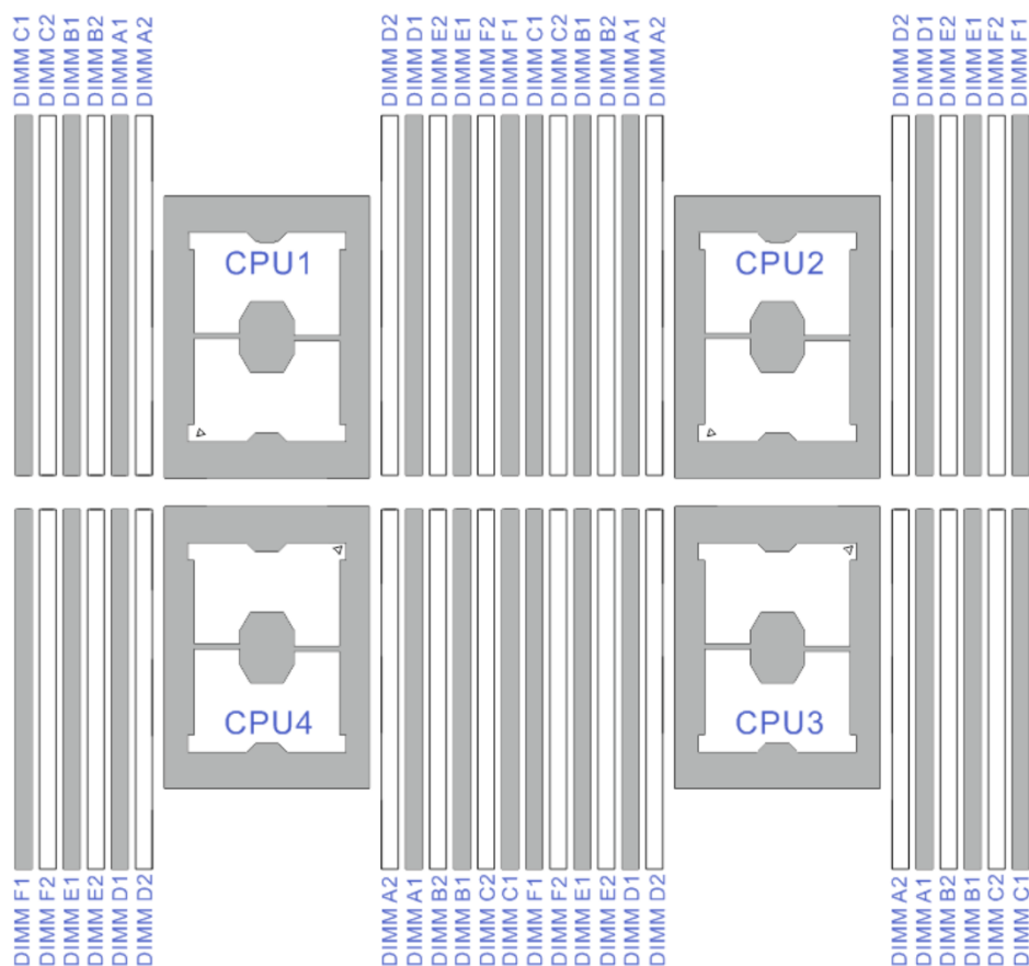
内存位号分页图示
